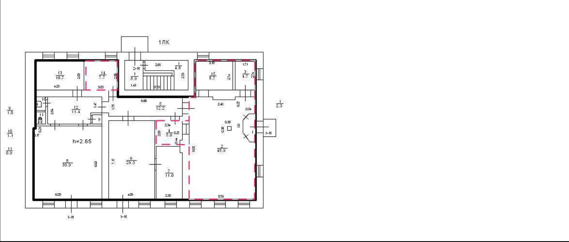
План 1 этажа
