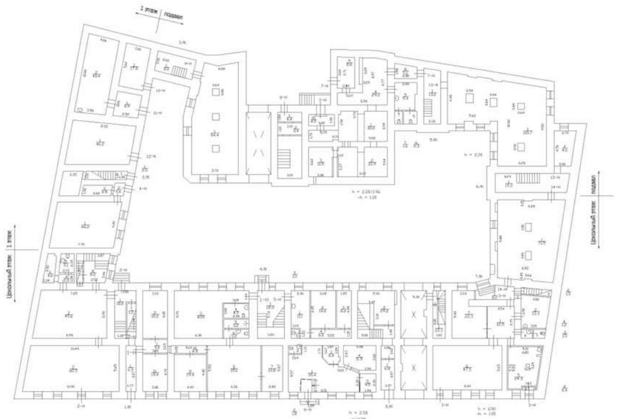
План подвала и 1 этажа
