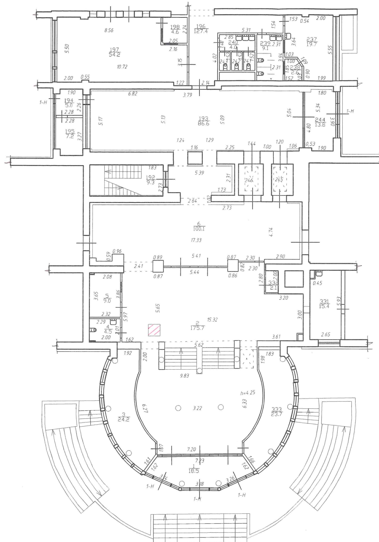
План части 1 этажа
