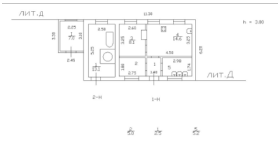
Рисунок 14. План 1 этаж литера Д
