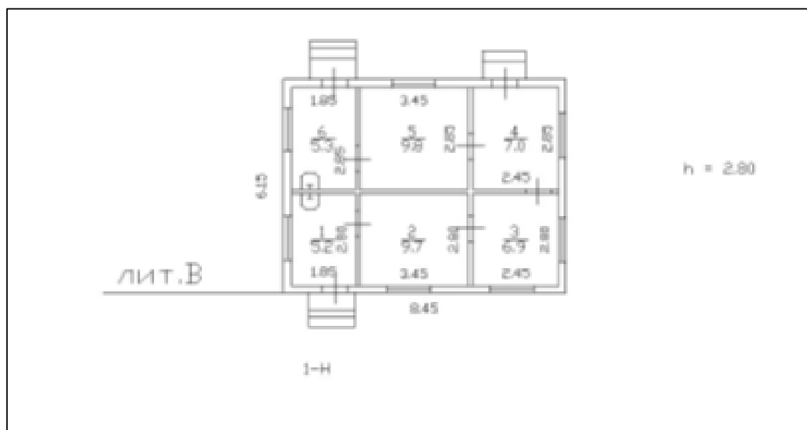
Рисунок 13. План 1 этаж литера В
