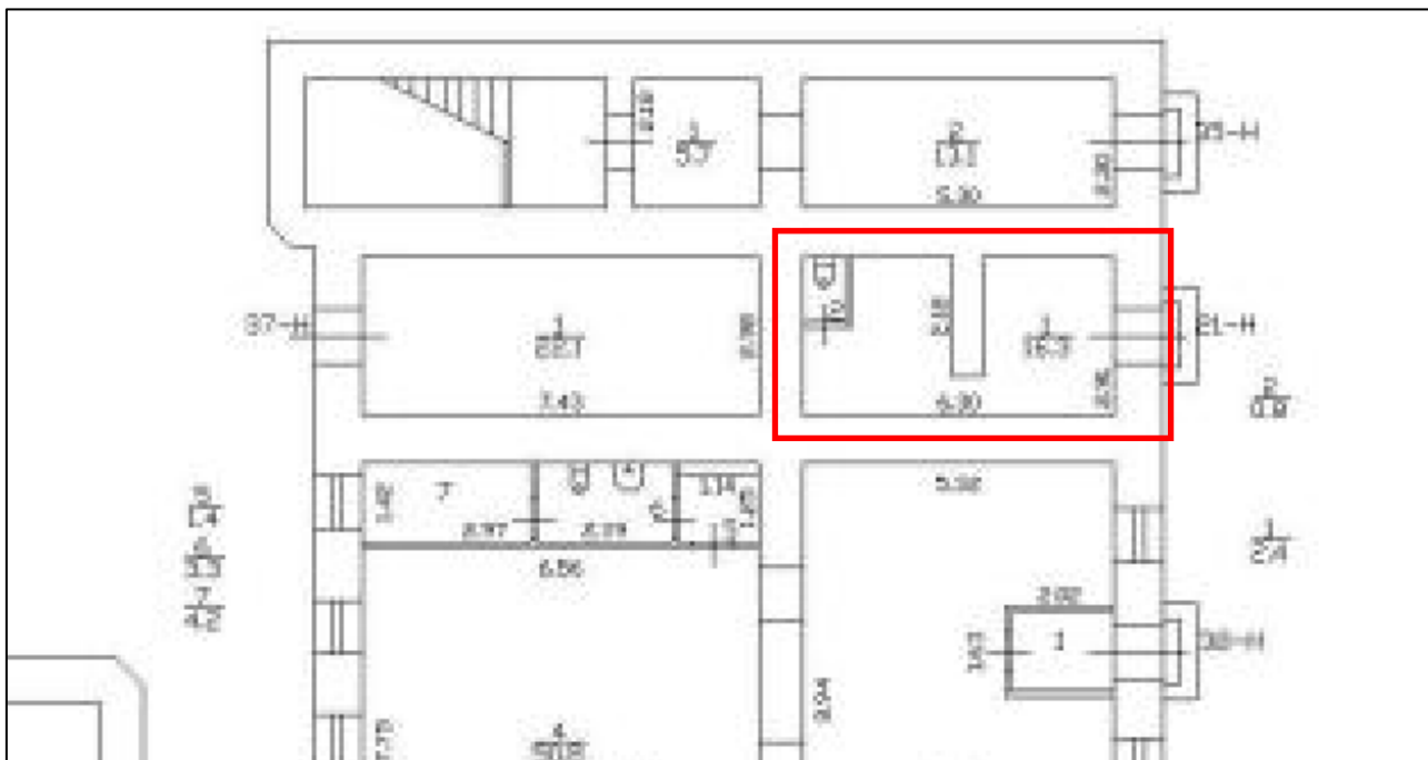
Рис. 3. План помещения
