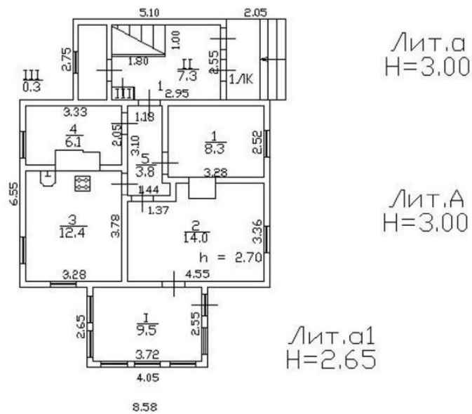
Рисунок 2. План 1-го этажа.
