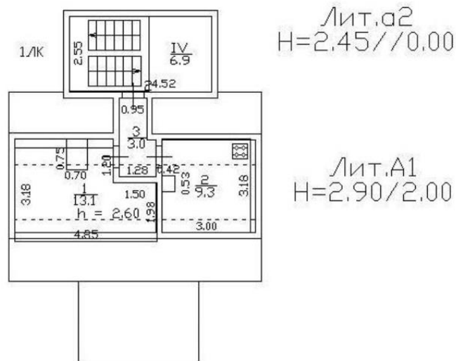
Рисунок 3. План мансарды.
